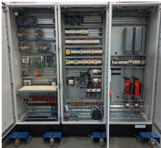
Beispiel eines Steuerschranks mit DataView Full Retrofit
